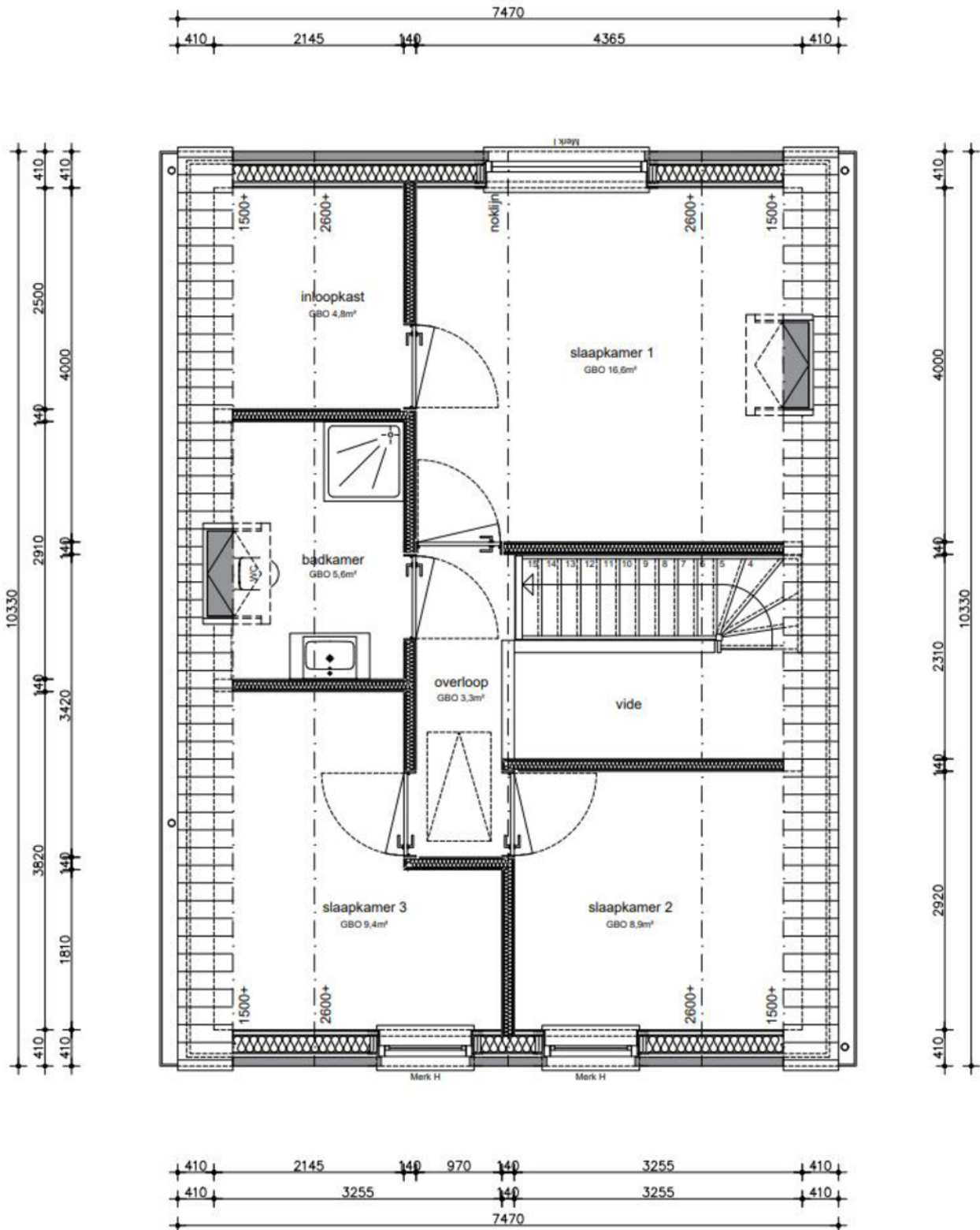
Verdieping 1:50
